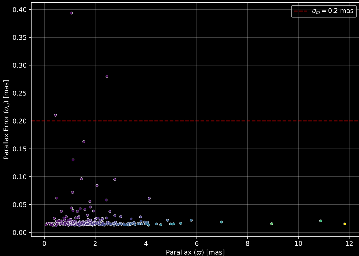
GALAH DR4 Field: [617] Parallax Quality (n= 299)
