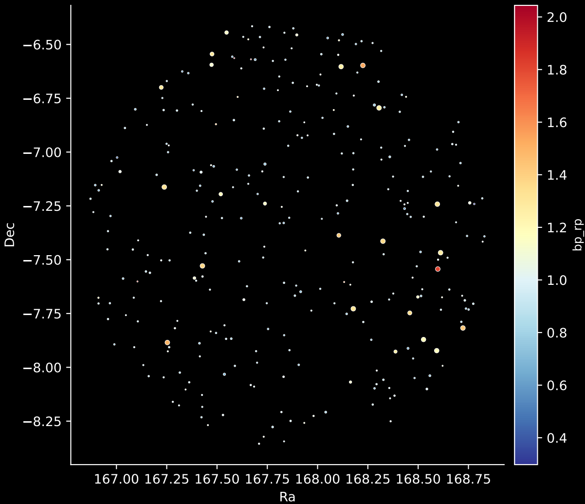
GALAH DR4 Field: [617] Stars: 299
