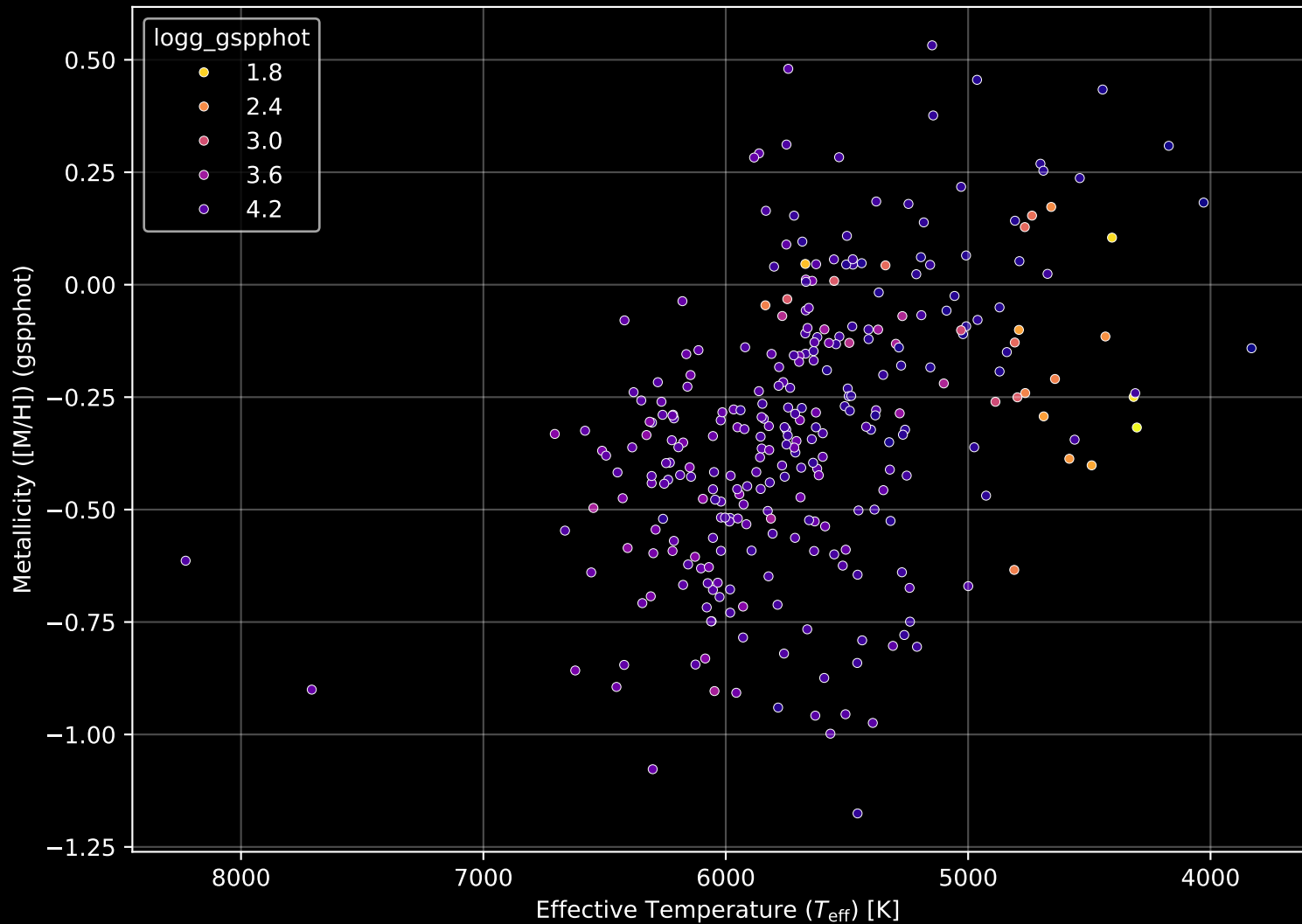
GALAH DR4 Field: [617] Stellar Population Parameters (n= 299)
